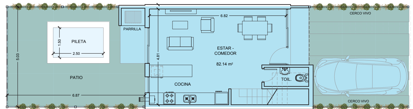
Planta baja tipo
