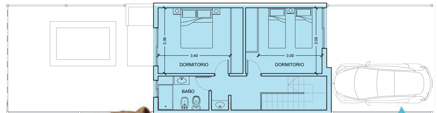
Planta alta tipo
